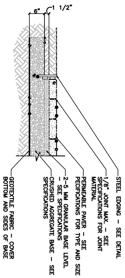
SECTION N.T.S.
